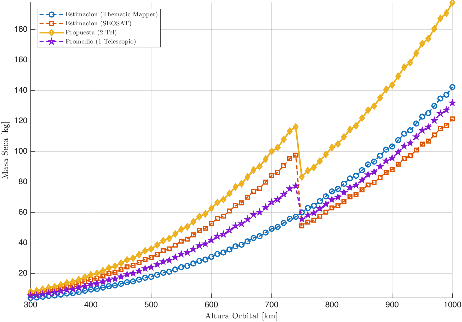
Comparativa de Masa Seca vs. Altura Config: 1 Sat, 2 Tel, Det 1, Cassegrain
